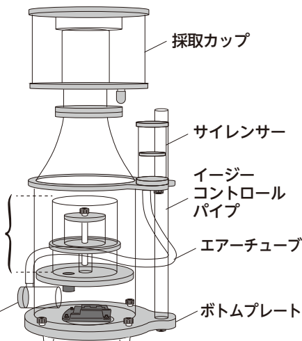
ポンプ 吸水口パーツ
